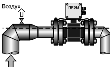
Рисунок 9 – Установка ПРЭМ в верхней точке трубопровода
